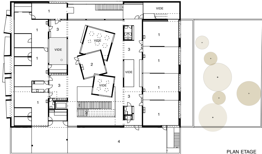
PLAN ETAGE
