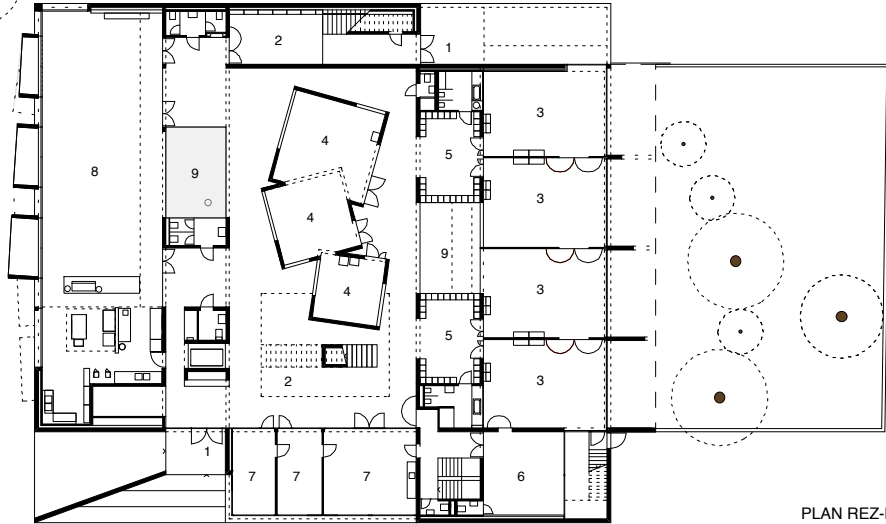
PLAN REZ-DE-CHAUSSEE
