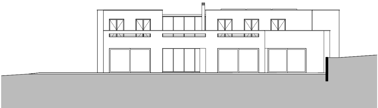
elevation sud
