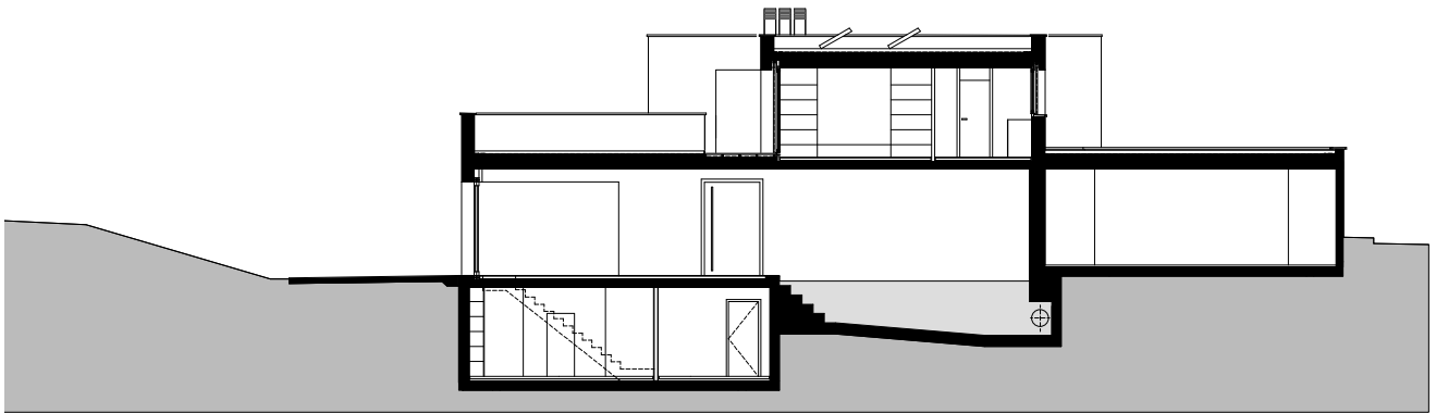
coupe BB
