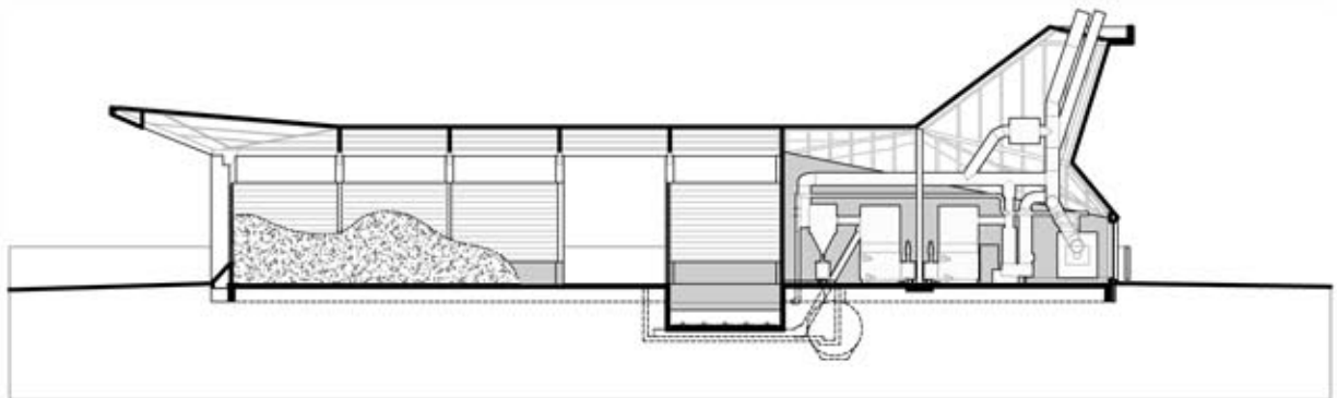
Coupe longitudinale
