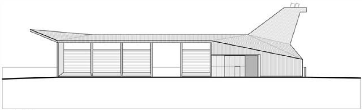
Façade Sud
