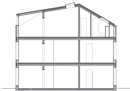
Coupe transversale 1:200
