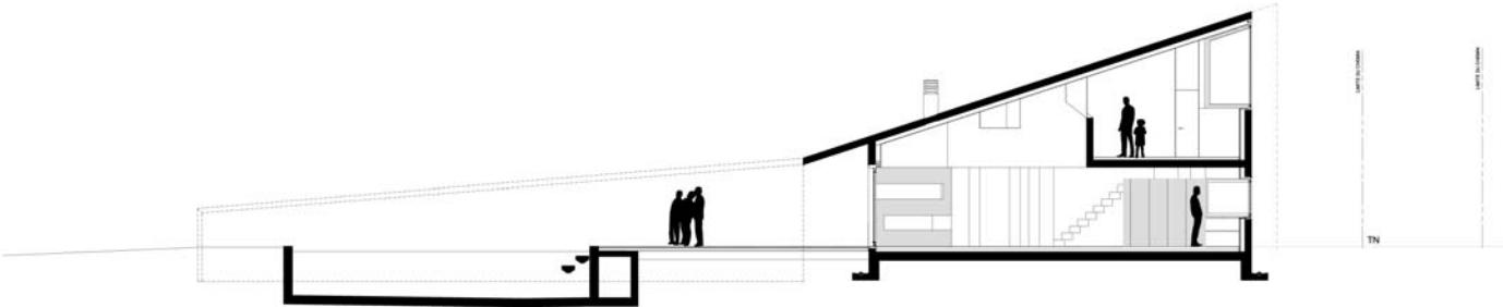
COUPE LONGITUDINALE
