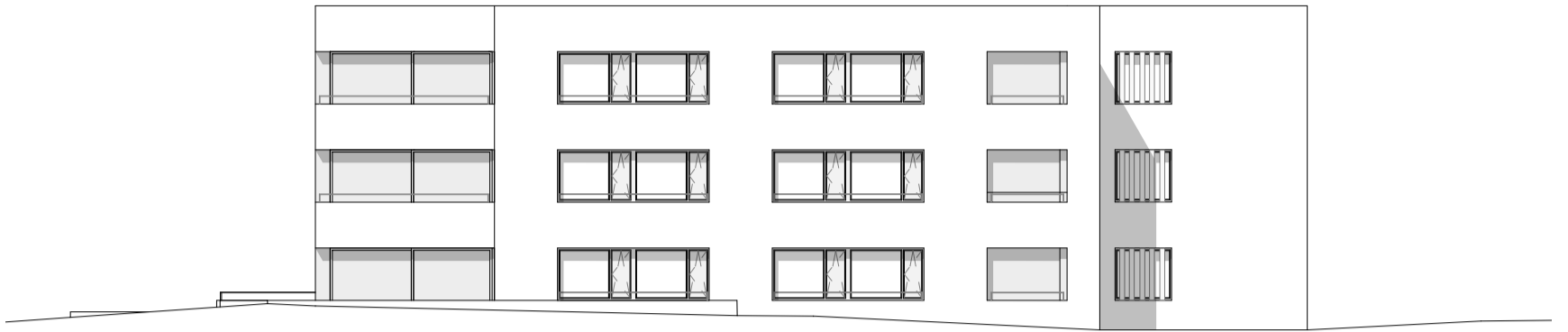
élévation est
