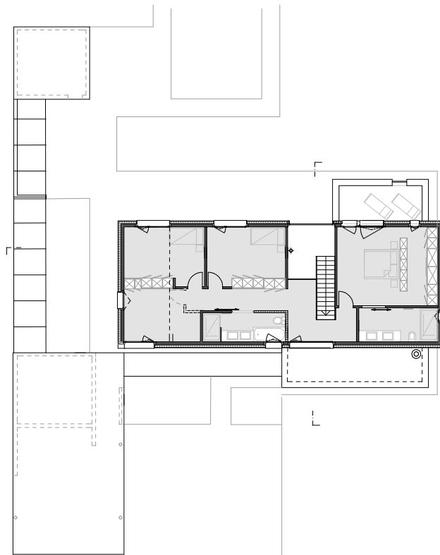
Etage
