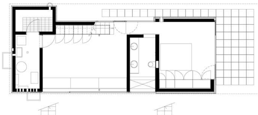
PLAN SOUS-SOL
