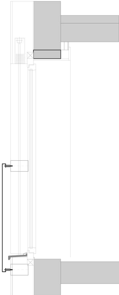
Détail garde-corps
