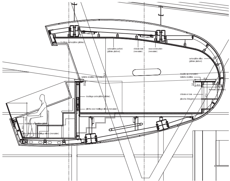
Coupe transversale dans les loges
