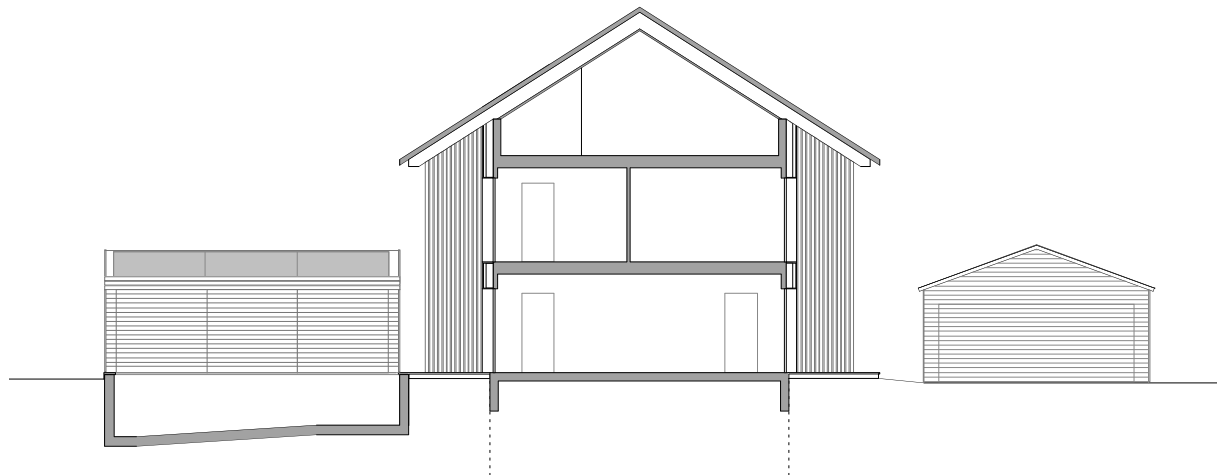
coupe AA 1/200
