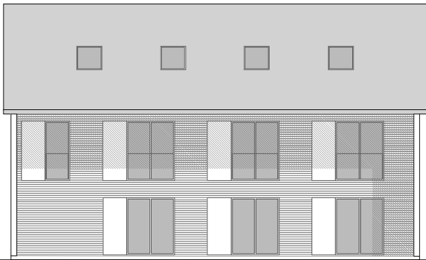
façade nord-ouest 1/200
