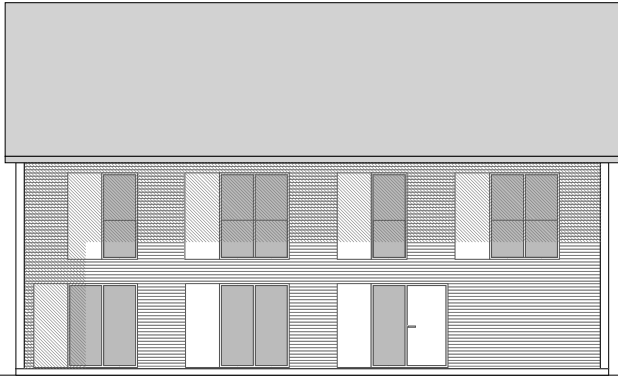
façade sud-est 1/200
