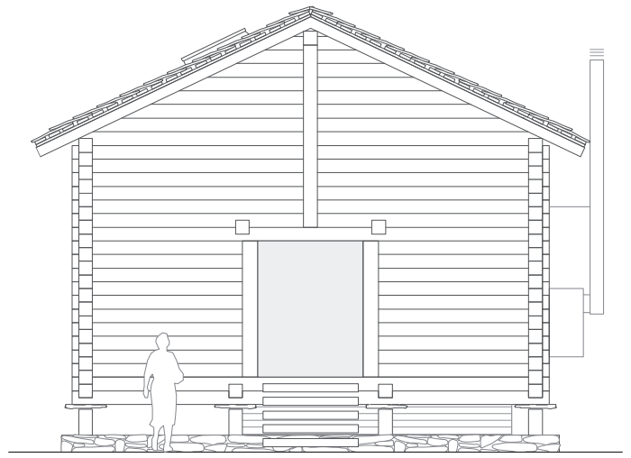
élévation est
