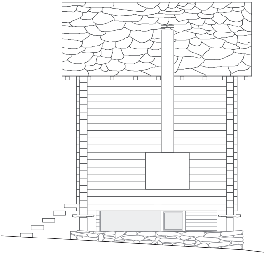
élévation nord
