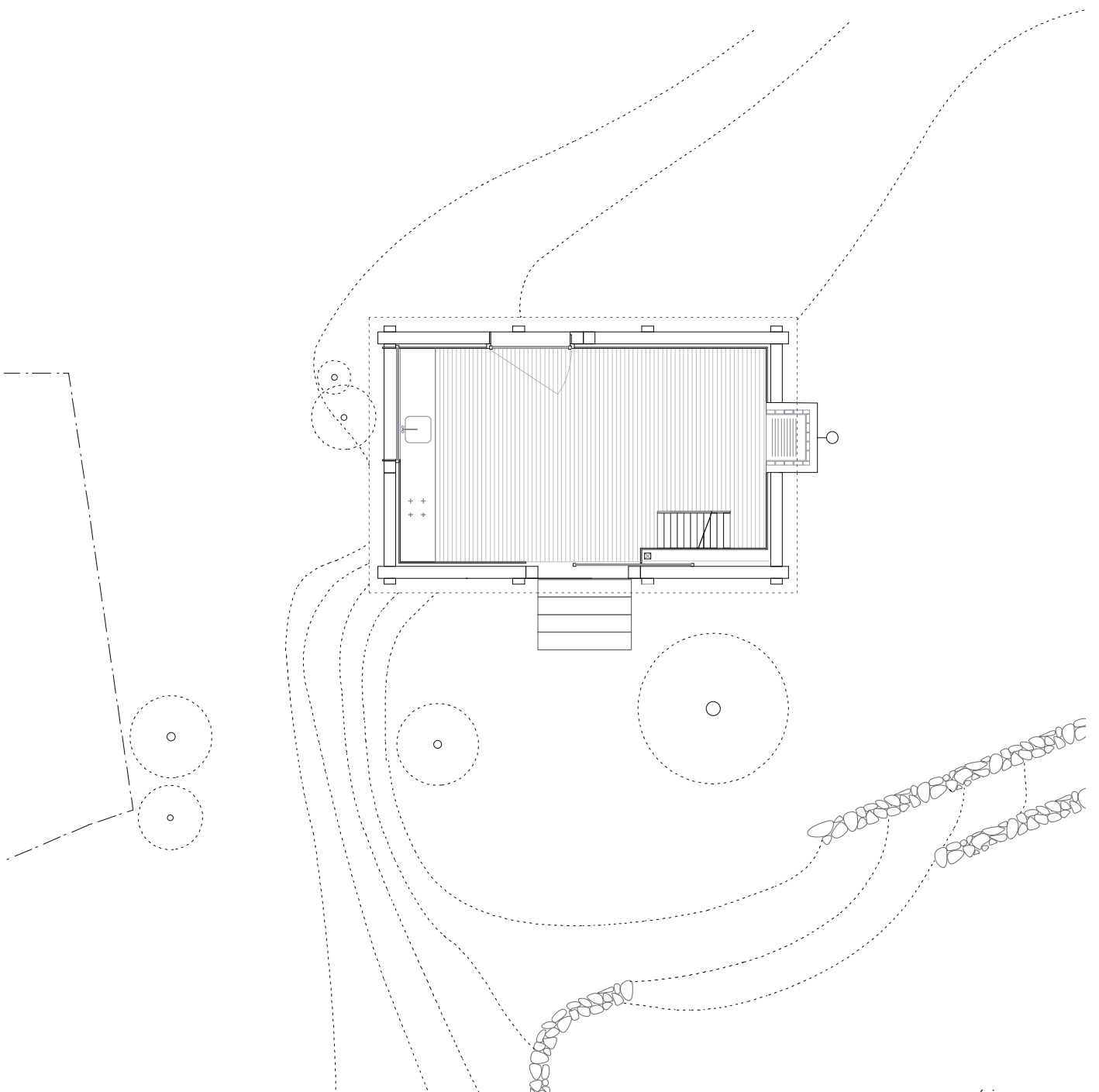
rez supérieur
