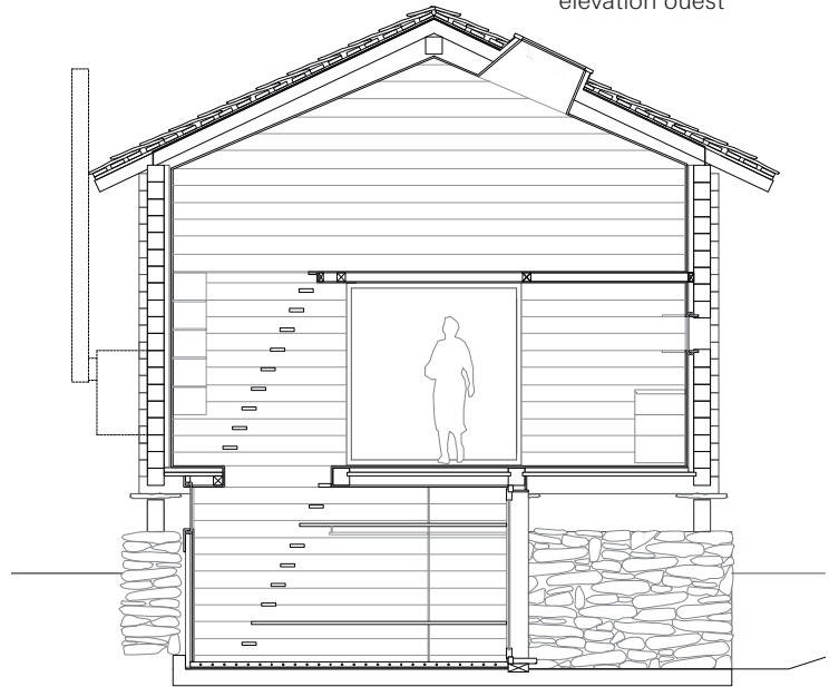
coupe
