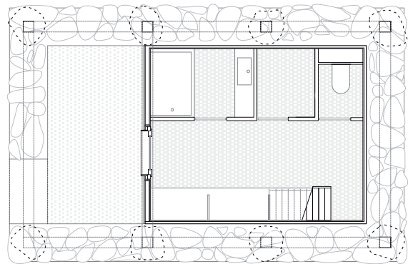
rez inférieur
