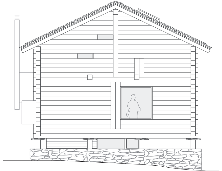
élévation ouest
