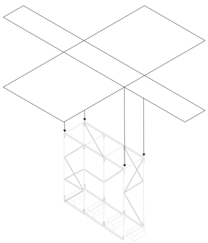
SCHÉMAS PLATEAU INFÉRIEUR ET EMBOTTEMENT PIÈCES
