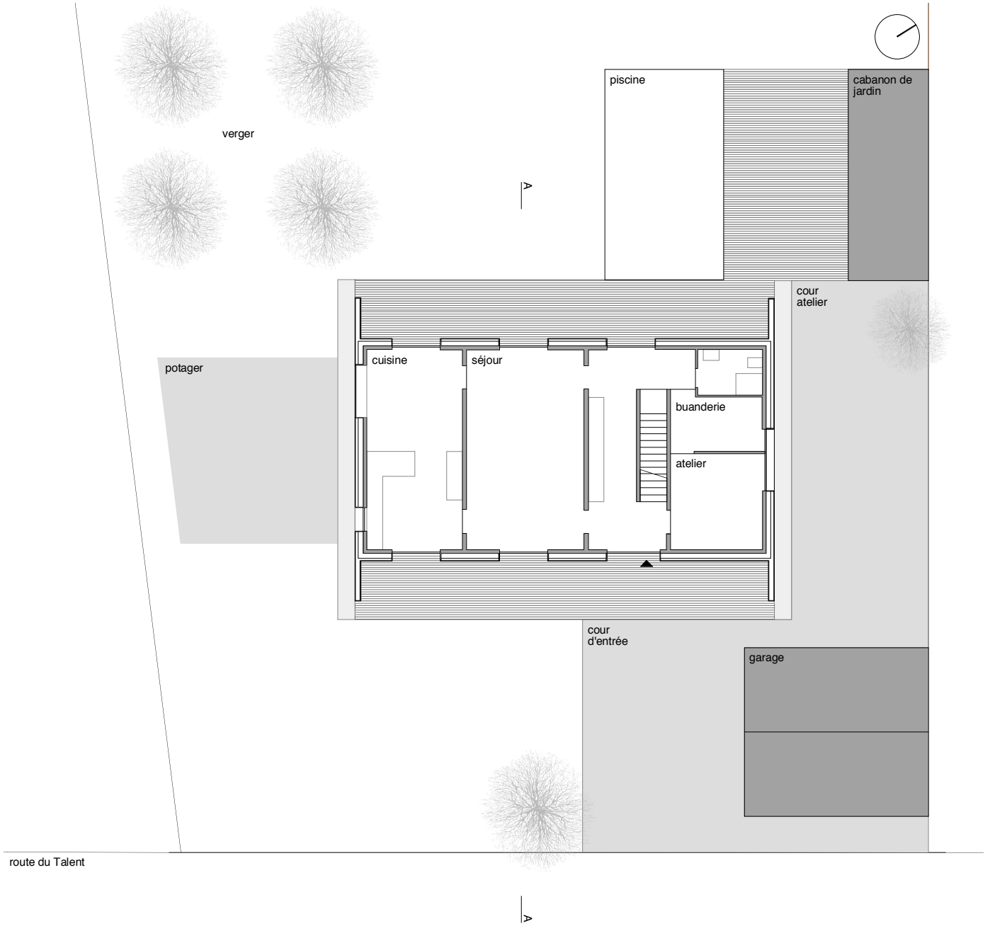
rez 1/200
