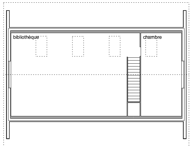
combles 1/200
