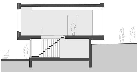
COUPE B-B
