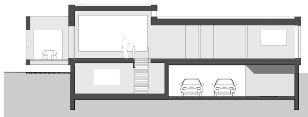
COUPE A-A
