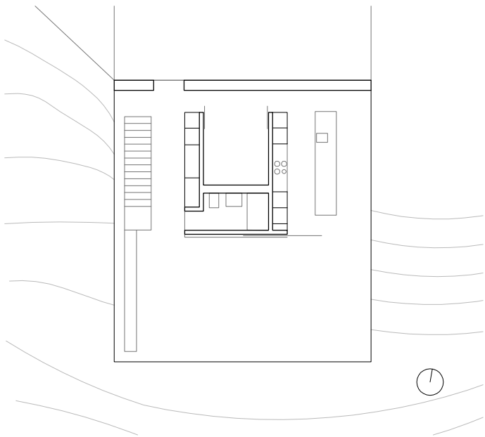
Rez supérieur
