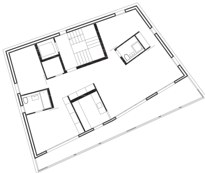
Plan d'étage type 1:200
