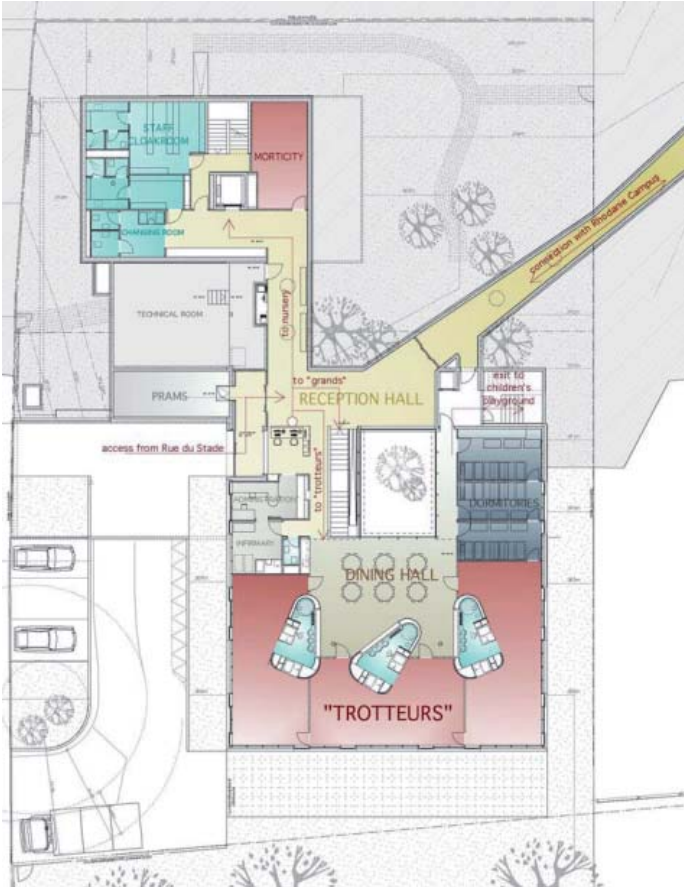
Plan niveau 00
