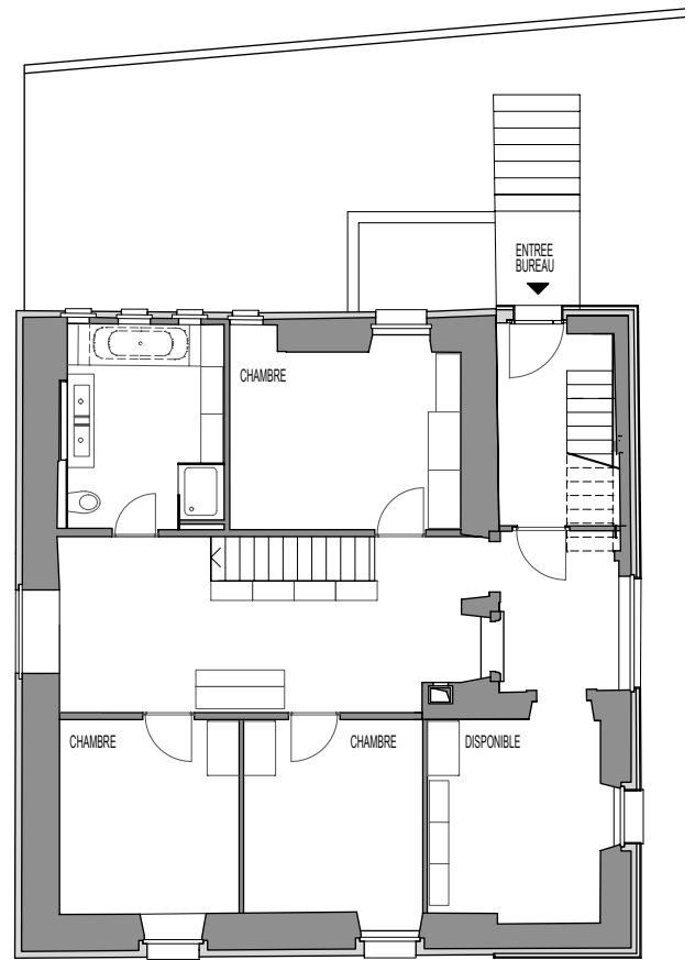
REZ-DE-CHAUSSEE SUPERIEUR
