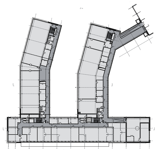
Plan étage
