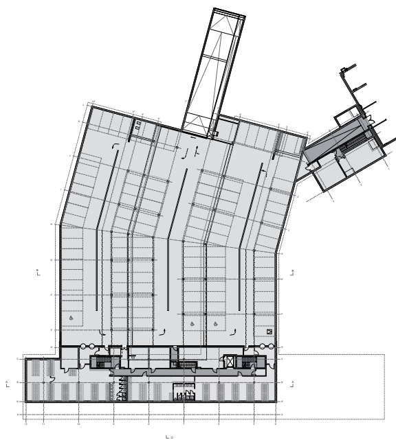
Plan sous-sol
