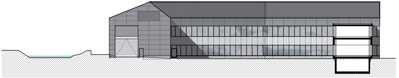
Façade Sud
