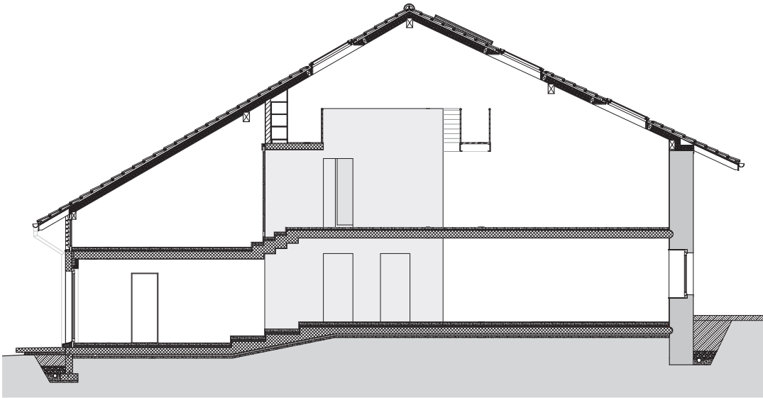
COUPE LONGITUDINALE
