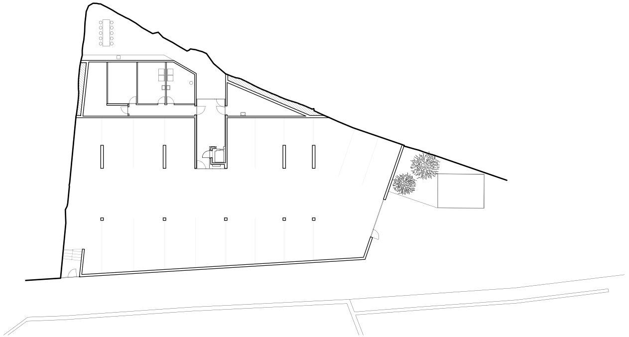
niveau 0 parking
