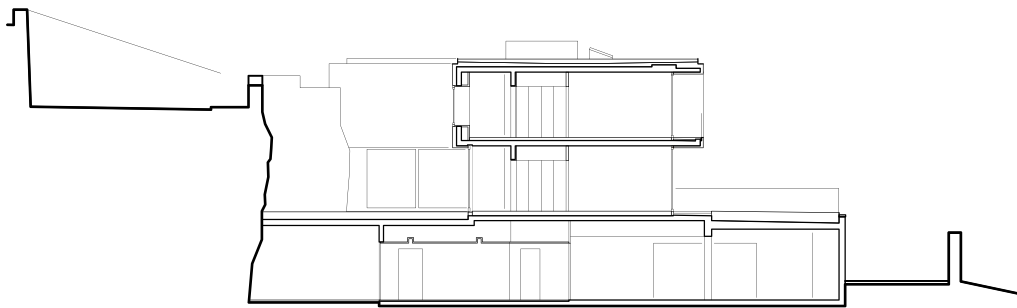
coupe transversale
