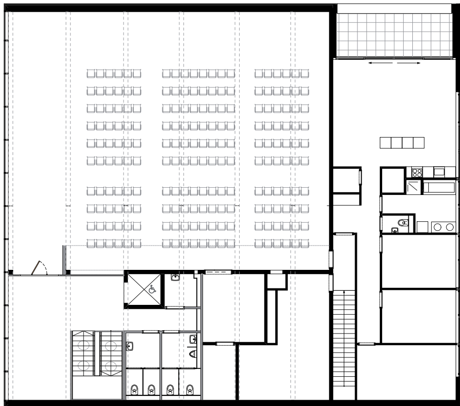
Plan étage
