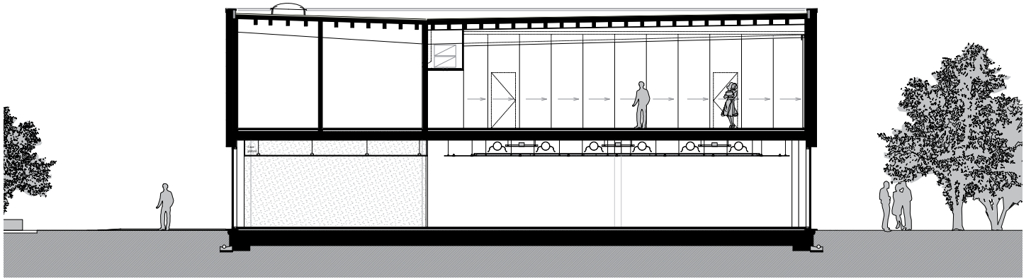
Coupe 1
