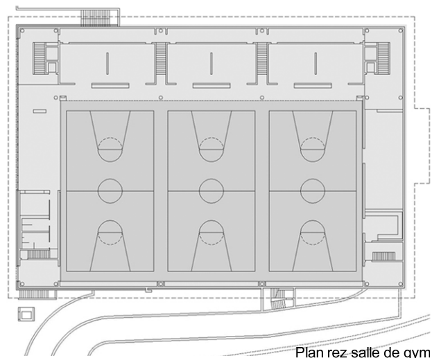
Plan rez salle de gym
