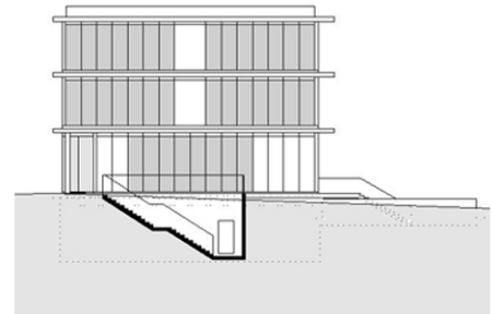
Coupe crèche
