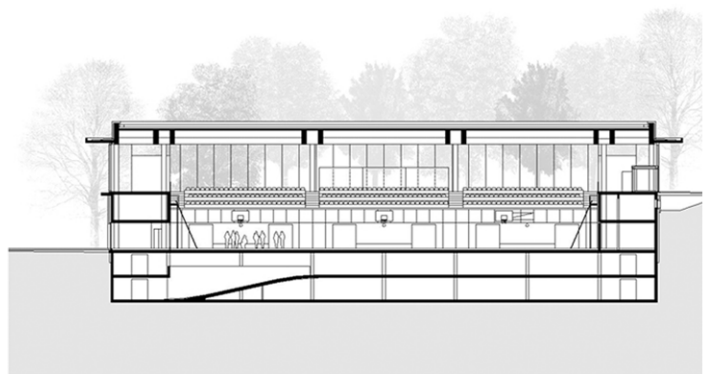
Coupe salle de gym
