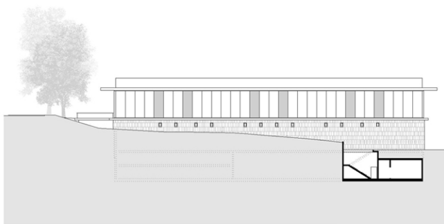
Façade salle de gym
