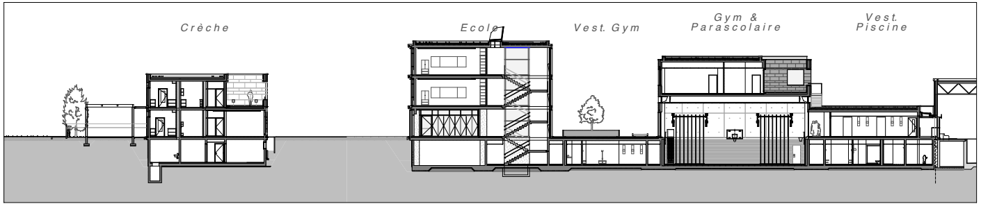
Coupe transversale
