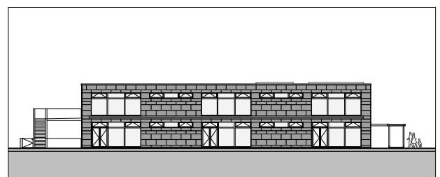
Élévation crèche
