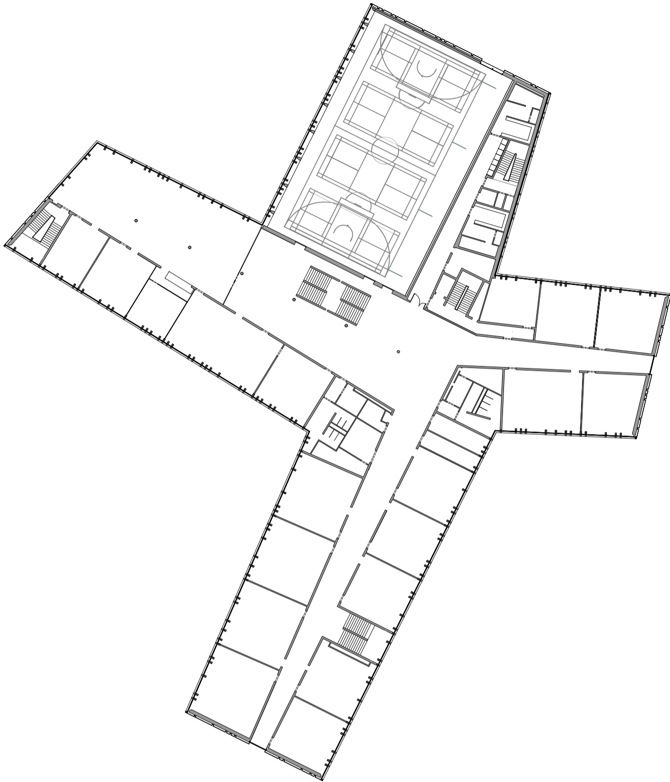
plan du 2 ème étage
