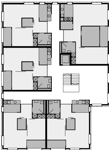
étages types
